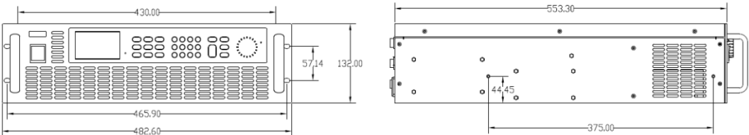
3U机型尺寸图
