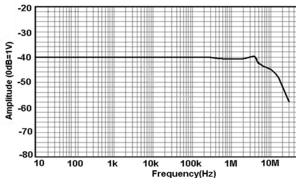
图 16 HCP8500 幅频曲线
