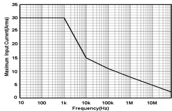
图 2.b HCP8030C 最大测量电流 VS 频率曲线
