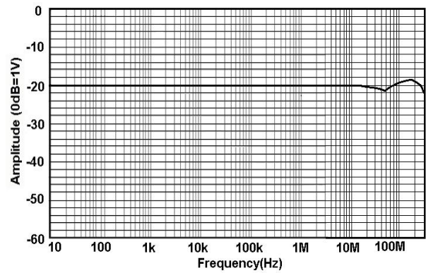
图 1.d HCP8030H 幅频曲线
