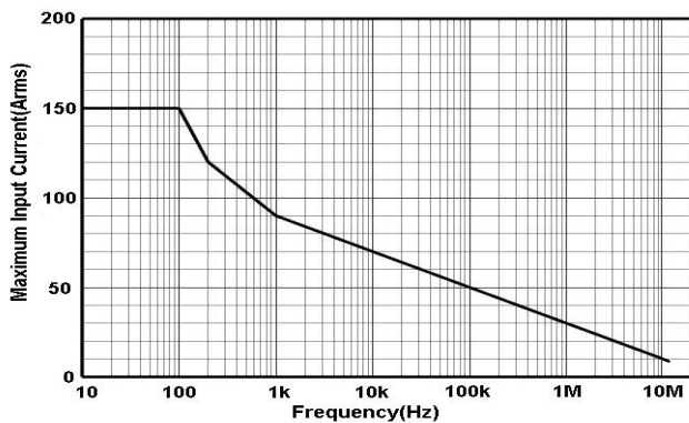
图 11.a HCP8150 最大测量电流 VS 频率曲线 (超过该曲线所示最大电流连续使用会导致探头烧毁)
