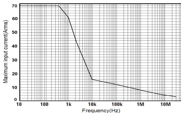
图 8 HCP8070 最大测量电流 VS 频率曲线 (超过该曲线所示最大电流连续使用会导致探头烧毁)
