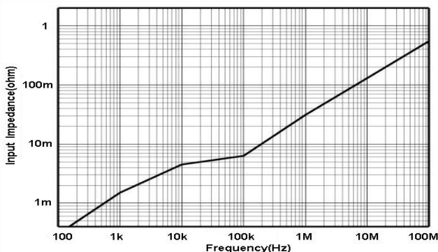
图 3.c HCP8030D 输入阻抗 VS 频率曲线
