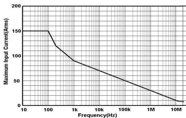
图 11.b HCP8150A 最大测量电流 VS 频率曲线 (超过该曲线所示最大电流连续使用会导致探头烧毁)
