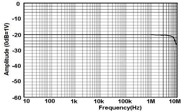
图 13 .b HCP8300A 幅频曲线
