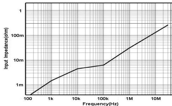
图 9 HCP8070 输入阻抗 VS 频率曲线
