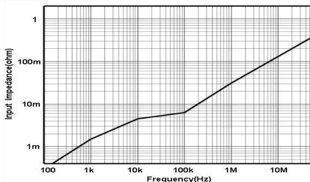
图 3.a HCP8030 输入阻抗 VS 频率曲线
