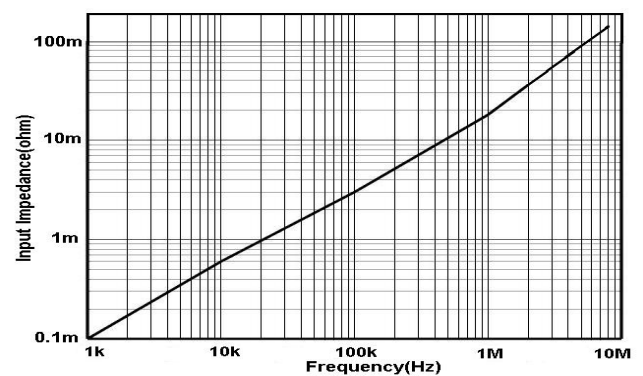
图 15.b HCP8300A 输入阻抗 VS 频率曲线
