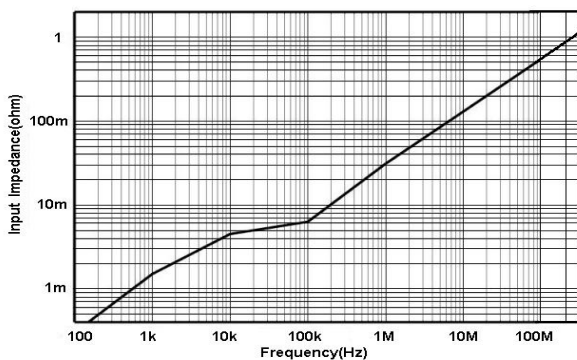
图 3.d HCP8030H 输入阻抗 VS 频率曲线
