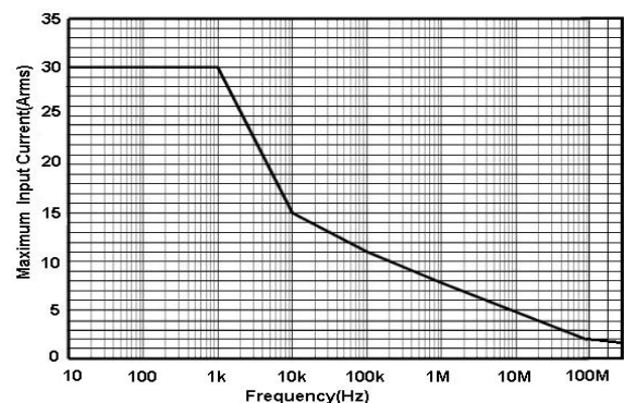
图 2.d HCP8030H 最大测量电流 VS 频率曲线
