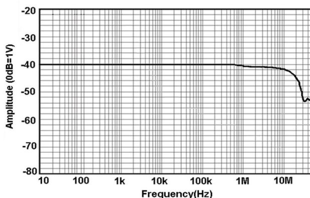
图 10.a HCP8150 幅频曲线
