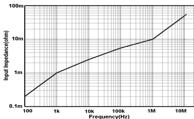
图 12.a HCP8150 输入阻抗 VS 频率曲线
