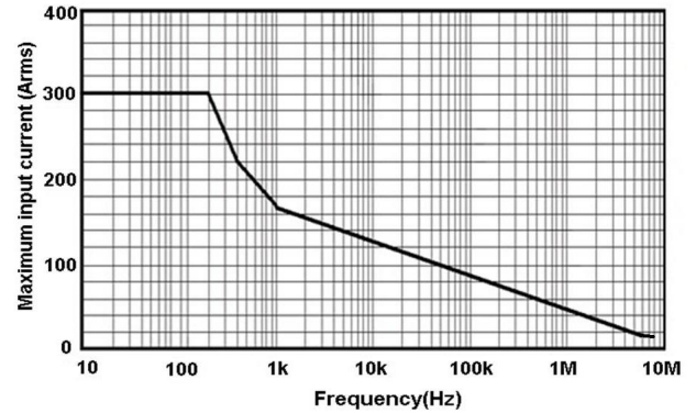
图 14.b HCP8300A 最大测量电流 VS 频率曲线 (超过该曲线所示最大电流连续使用会导致探头烧毁)
