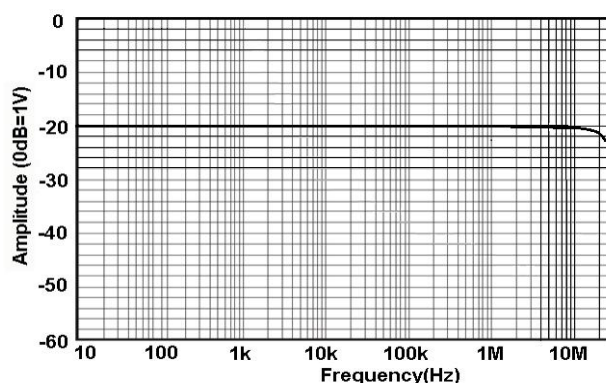
图 10.b HCP8150A 幅频曲线
