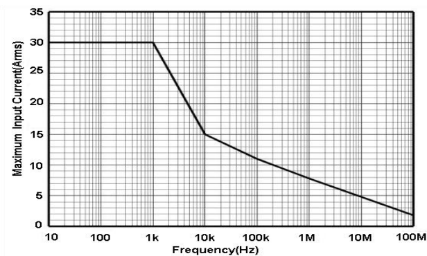
图 2.c HCP8030D 最大测量电流 VS 频率曲线
