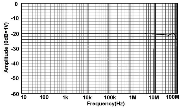
图 1.b HCP8030C 幅频曲线
