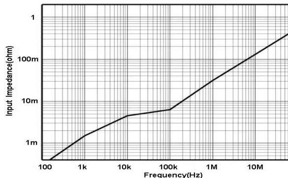
图 3.b HCP8030C 输入阻抗 VS 频率曲线
