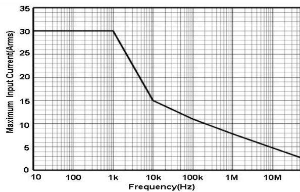
图 2.a HCP8030 最大测量电流 VS 频率曲线
