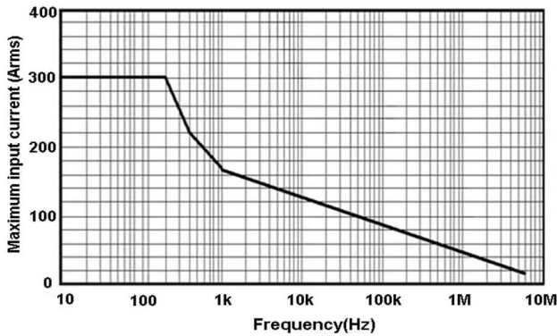
图 14.a HCP8300 最大测量电流 VS 频率曲线 (超过该曲线所示最大电流连续使用会导致探头烧毁)
