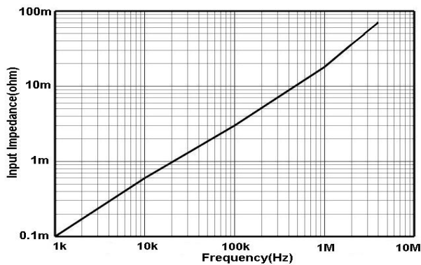
图 15.a HCP8300 输入阻抗 VS 频率曲线
