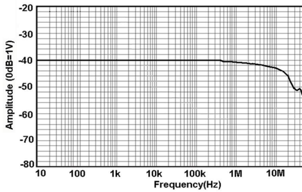
图 13.a HCP8300 幅频曲线
