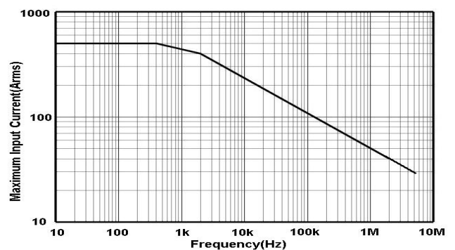
图 17 HCP8500 最大测量电流 VS 频率曲线 (超过该曲线所示最大电流连续使用会导致探头烧毁)
