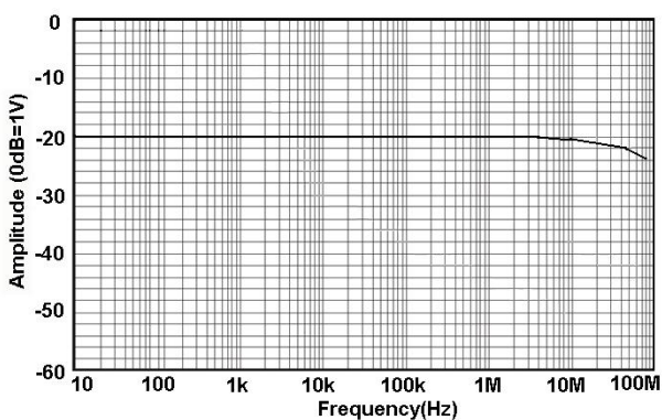
图 4 HCP8050 幅频曲线
