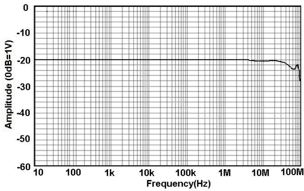
图 1.a HCP8030 幅频曲线
