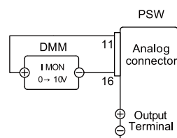
外部DMM监控输出电流
