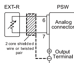
外部电阻控制电压输出
