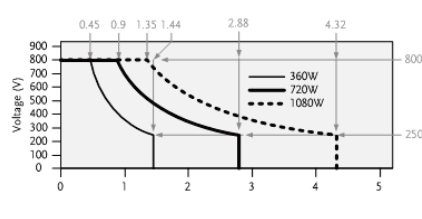
PSW 800V 系列工作区
