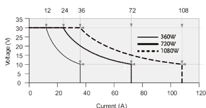
PSW 30V 系列工作区
