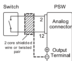
外部开关控制总电源断电
