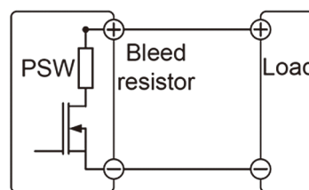
PSW-系列内置泄放电阻
