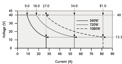
PSW 40V 系列工作区
