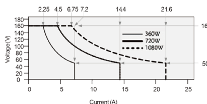
PSW 160V 系列工作区
