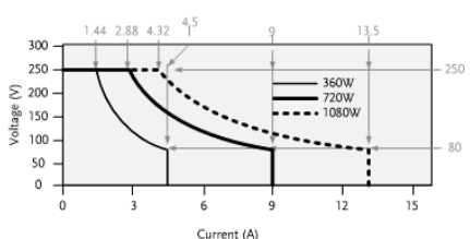
PSW 250V 系列工作区
