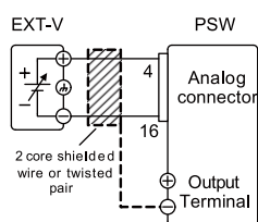
外部电压控制电压输出
