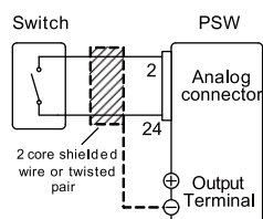
外部开关控制输出On/Off
