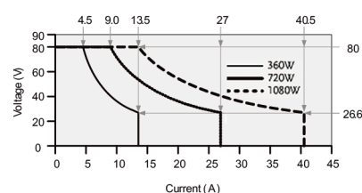
PSW 80V 系列工作区
