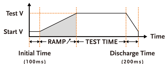
一个测试周期内输出电压可调
