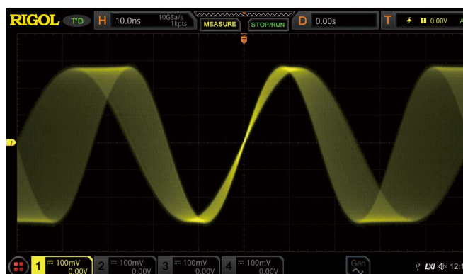
高刷新率模式下扫频信号每一帧的波形变化清晰可见
