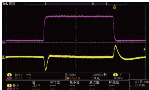
2台 IT6006B-500-40并机 设定电压:100V, 设定电流:56A 负载电流:60A
