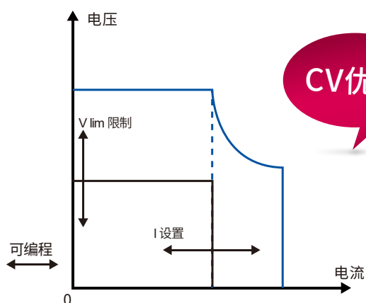
启动浪涌电流超电流量程, 高速建立电压 (CV-High, CC-Low, CV优势)
